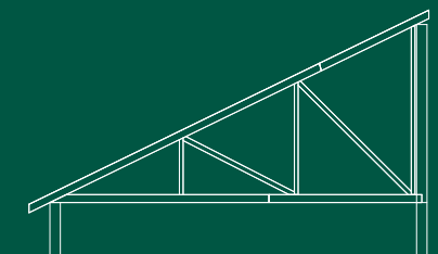
Ferme monopente de combles perdues
