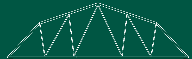
Ferme de combles perdus à facettes
