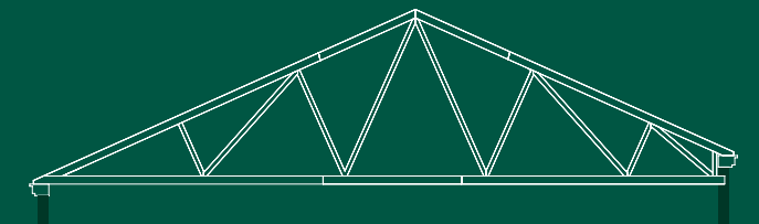
Ferme de combles perdues en double W tronquée à une extrémité
